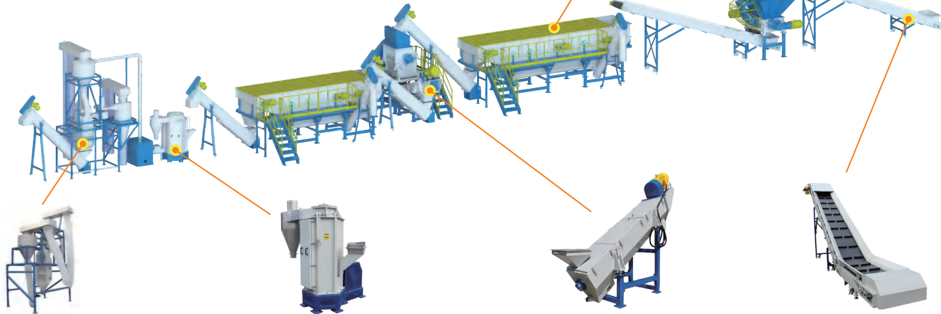
风选系统 Air Classifier 风送集料 Cyclone Collection 高效分离出灰尘和标签，收集成品物料。 Removes dirt and labels. Collects target materials.
